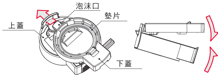
⑤ 上下蓋蓋回還原。下蓋的泡沫口插入上蓋的洞，蓋上會有“卡”聲音。
